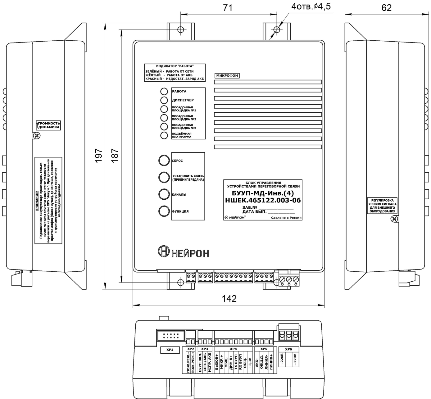
Рис.1 Внешний вид Блока управления устройствами переговорными «БУУП-МД-инв.(4)» НШЕК.465122.003-06
